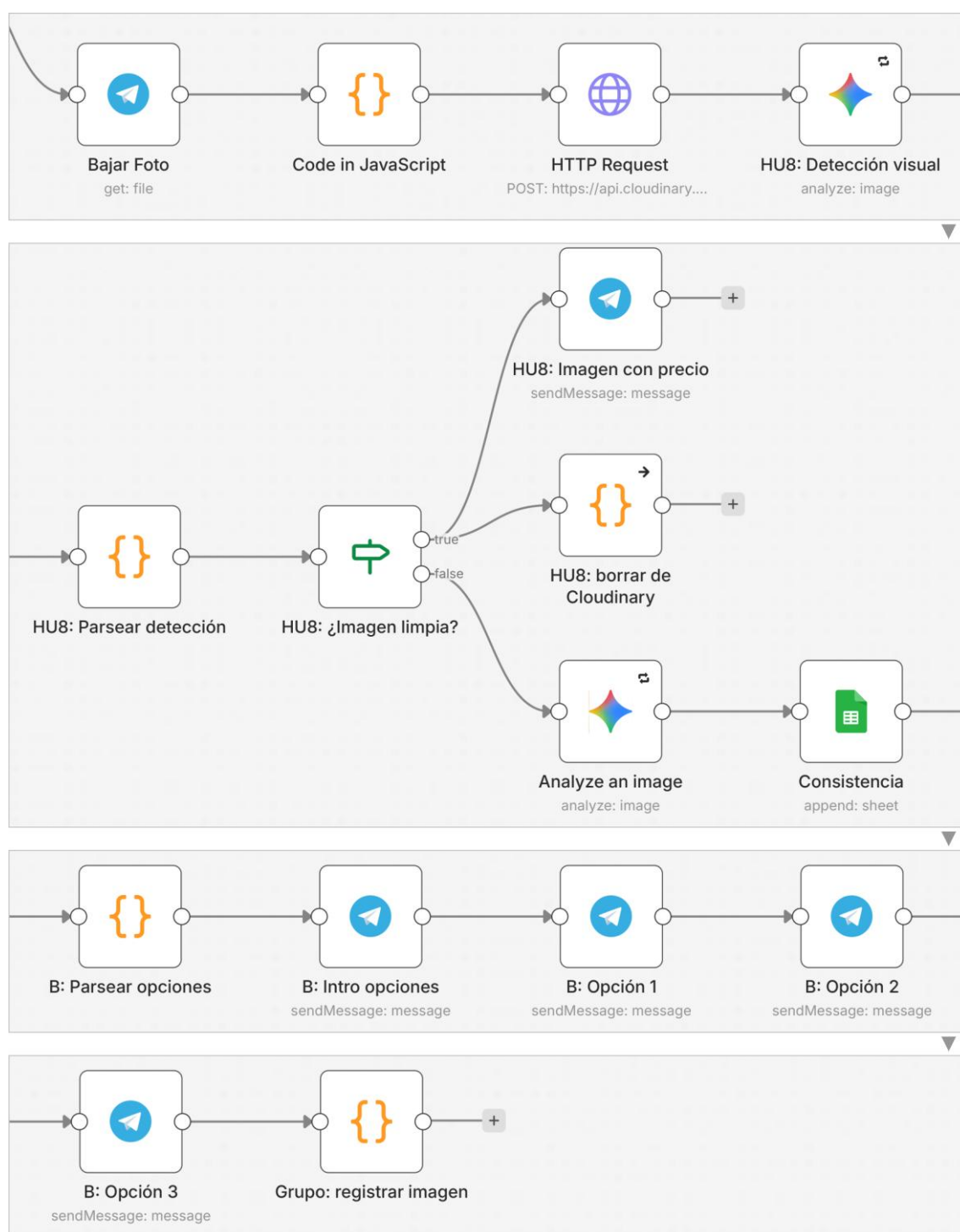
Figura 11. Rama de creación con imagen única en el workflow principal de n8n.
